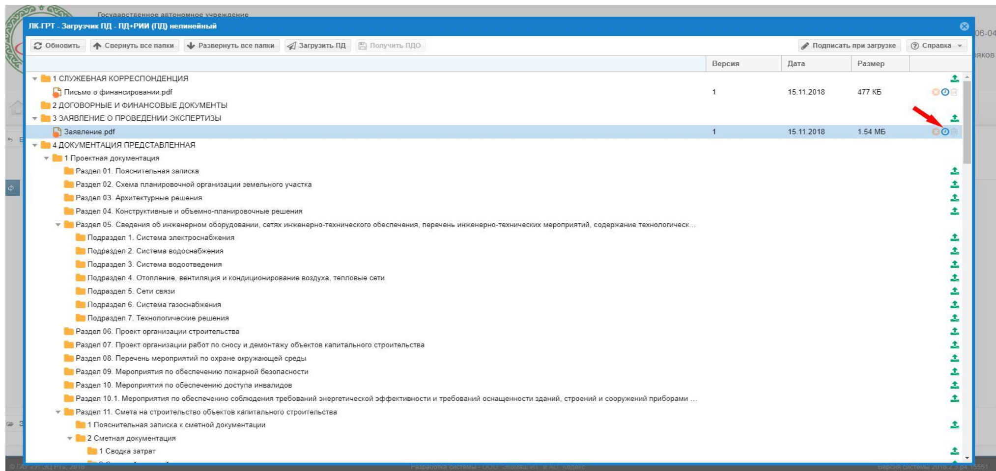
Скриншот 1
